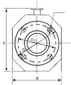
(DN15 DN80)
