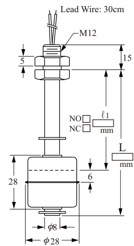
Washer: NBR
