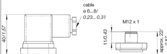
Cube plug DIN EN 175301-803 A (former DIN 43650)
